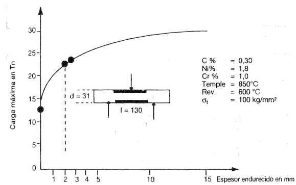
Figura 5: Influencia del espesor endurecido en la resistencia a flexión [1].
